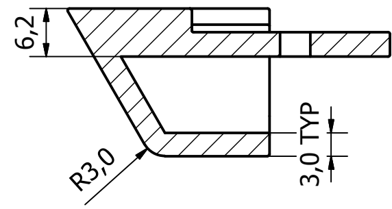
A-A ( 1.5:1 )
